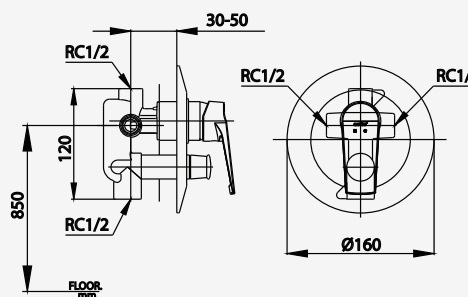
■ CT2249AV Concealed Mixer Stop Valve With Diverter วาล์วผสมเปิด-ปิดน้ำแบบก้านโยกชนิดฝังผนัง พร้อมตัวเปลี่ยนทิศทางน้ำ
