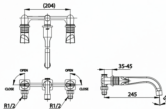
■ CT2283C46 3 Hole 8" Basin Mixer Faucet wall-mounted ก๊อกผสมอ่างล้างหน้า เซ็นเตอร์ 8 ชนิดติดตั้งผนัง
