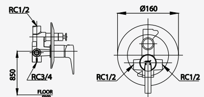
■ CT2267A Lever Handle Concealed Mixer Stop Valve with Diverter (2 Way) วาล์วผสมเปิด-ปิดน้ำก้านโยก ชนิดฟังก์ชัน พร้อมวาล์วเปลี่ยนทิศทางน้ำ (2 ทิศทาง)
