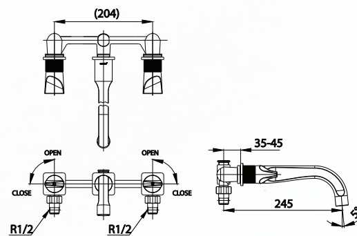
■ CT2283C45 3 Hole 8" Basin Mixer Faucet wall-mounted ก๊อกผสมอ่างล้างหน้า เซ็นเตอร์ 8 ชนิดติดตั้งผนัง
