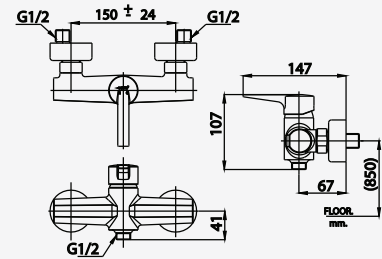
■ CT2264A Lever Handle Exposed Shower Mixer ก๊อกผสมขึ้นอาบนํ้าแบบก้านโยก
