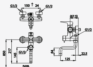
■ CT5102A Lever Handle Concealed Mixer Stop Valve with Diverter (3 Ways) ก๊อกผสมขึ้นอาบนํ้าพร้อมตัวก๊อกลงพื้น (เกลียวบน)
