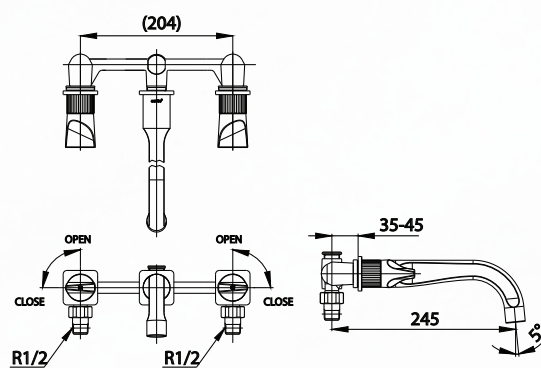
■ CT2283C44 3 Hole 8" Basin Mixer Faucet wall-mounted ก๊อกผสมอ่างล้างหน้า เซ็นเตอร์ 8 ชนิดติดตั้งผนัง
